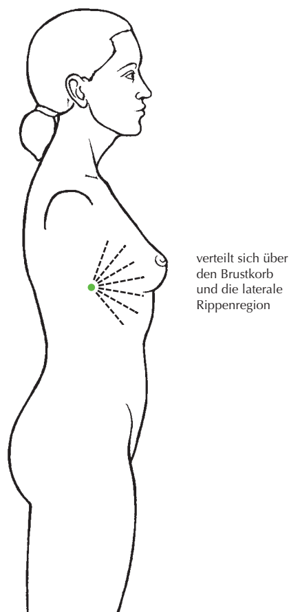
Abb. 2 Die große Milz-Verbindungsleitbahn
